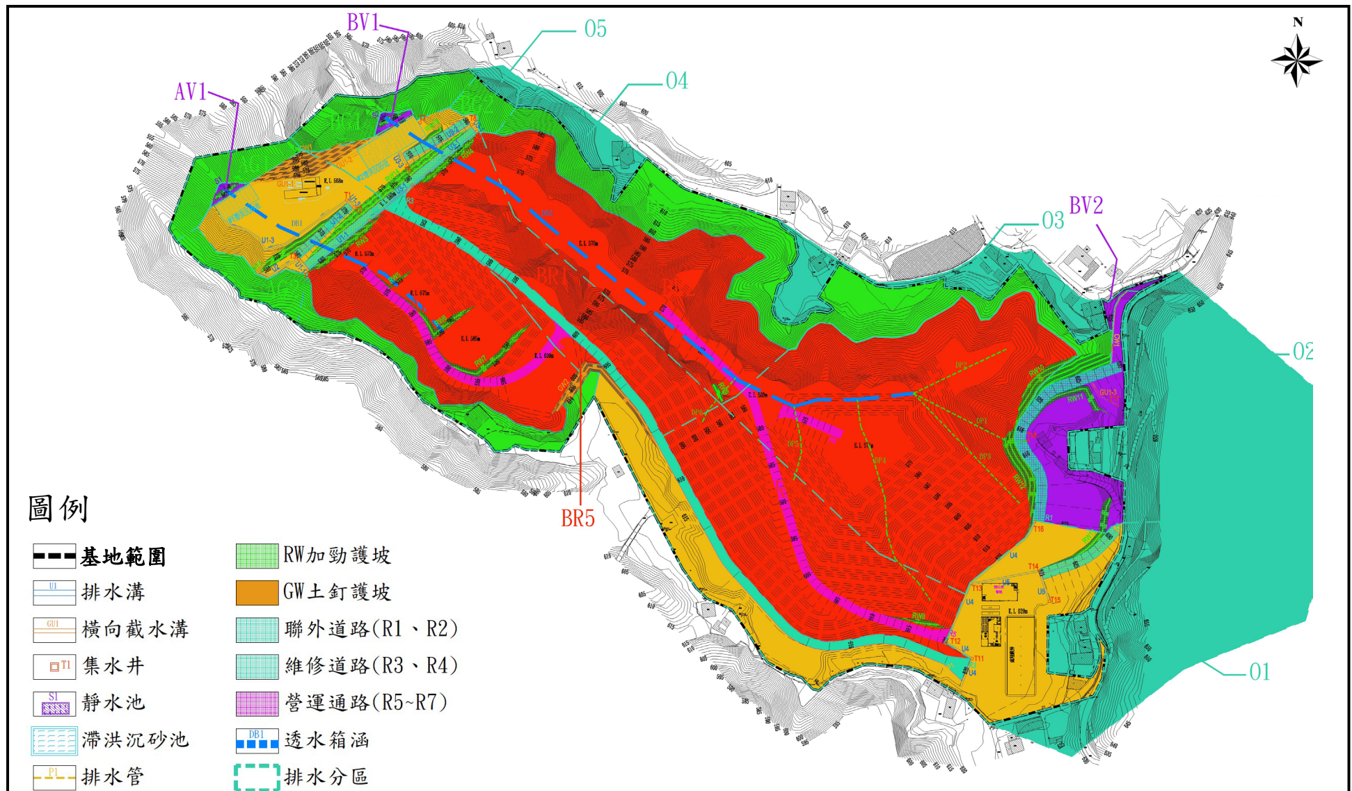
圖4-17 整地後掩埋前排水分區圖
