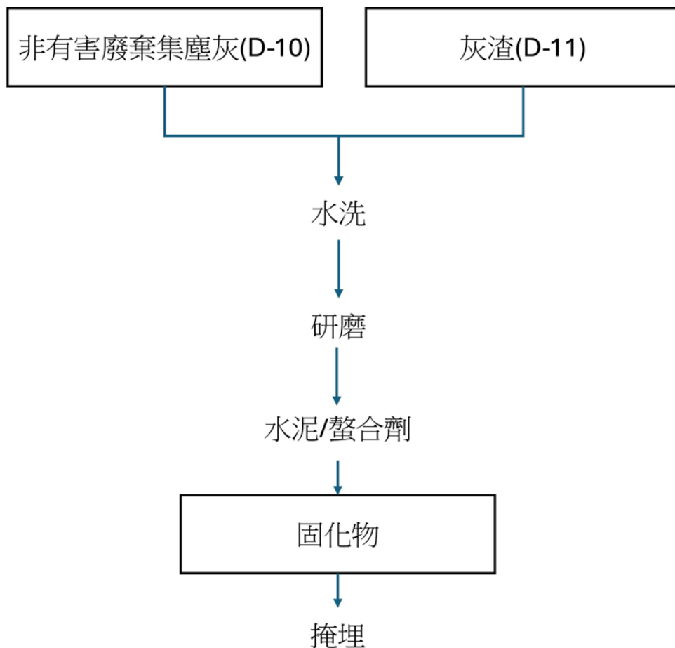
圖 4-9 固化流程示意圖
