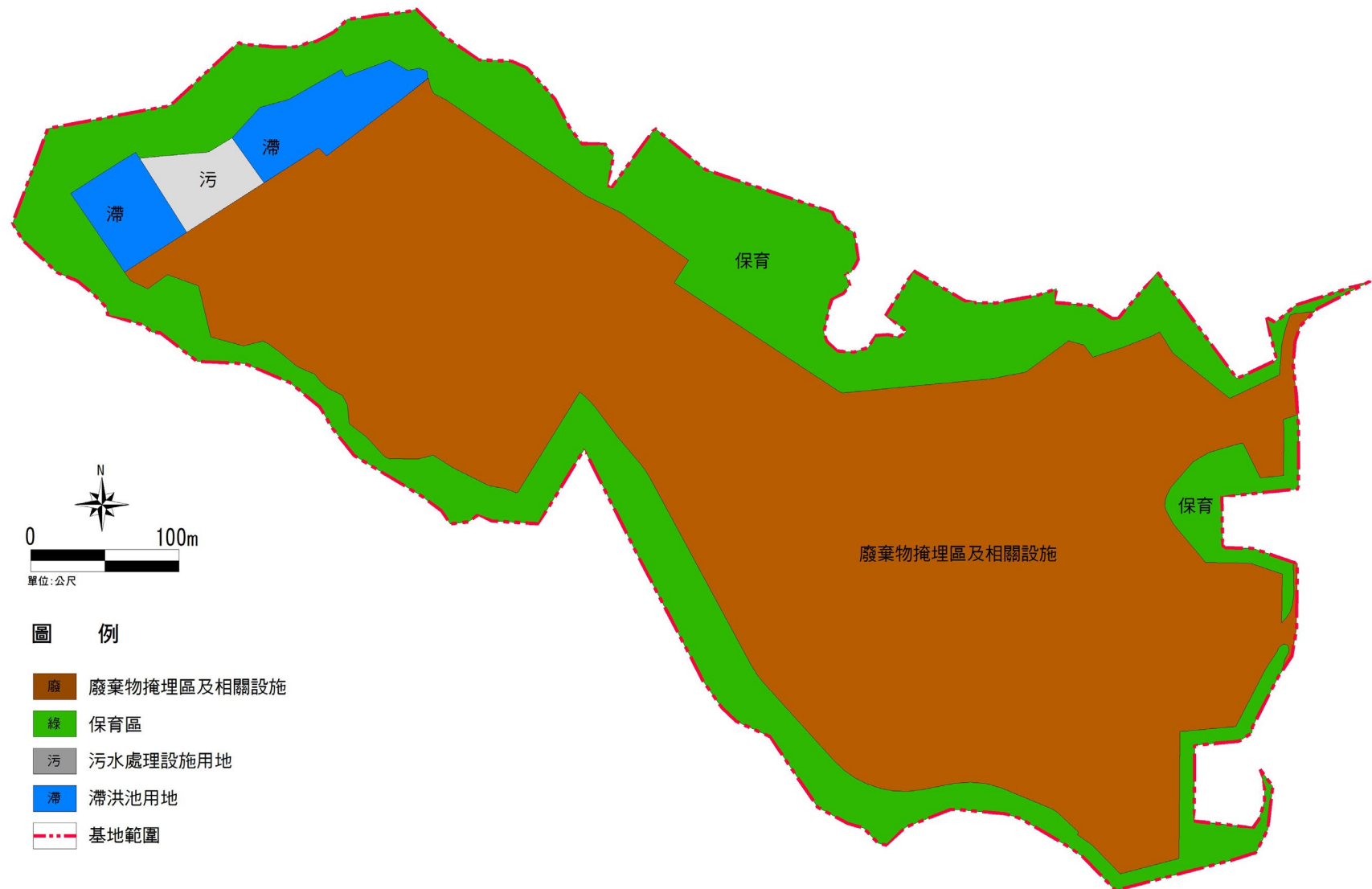
圖4-1 整復前土地使用計畫圖
