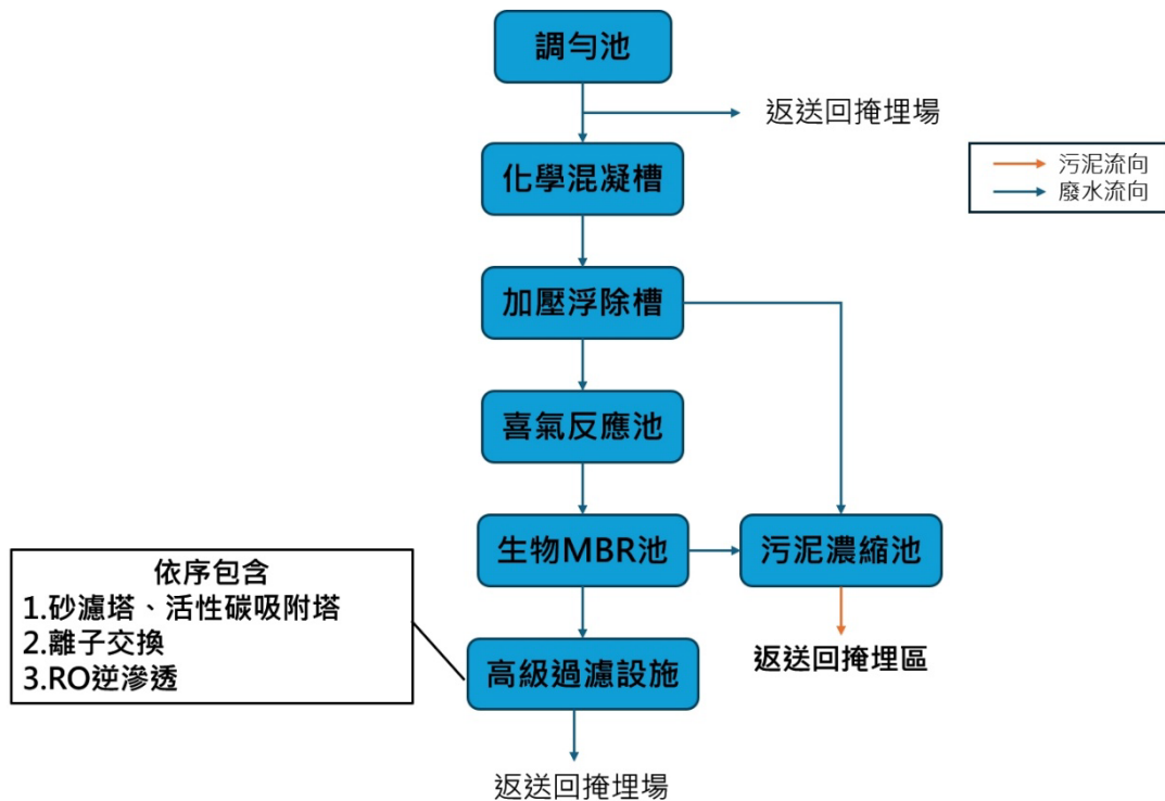
圖 5-1 廢污水處理流程圖
