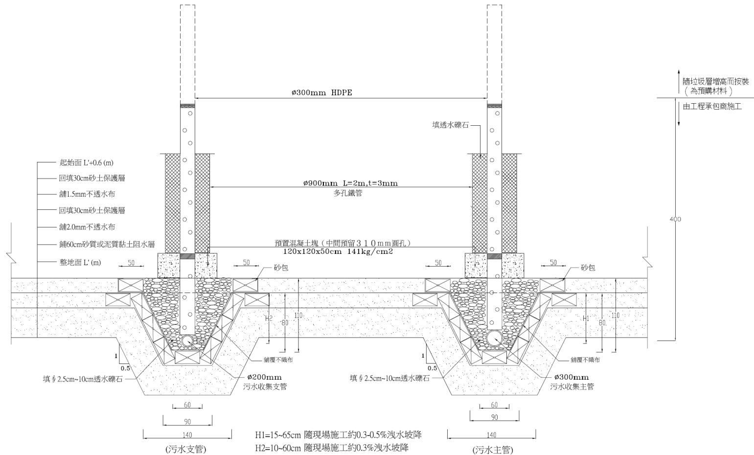
圖4-6 不透水及排水設施設計示意圖
