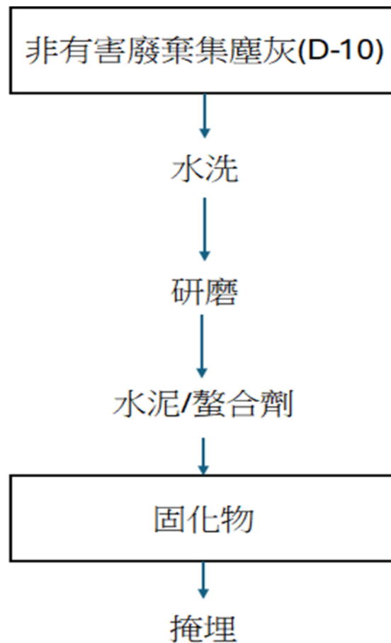
圖 4-9 固化流程示意圖
