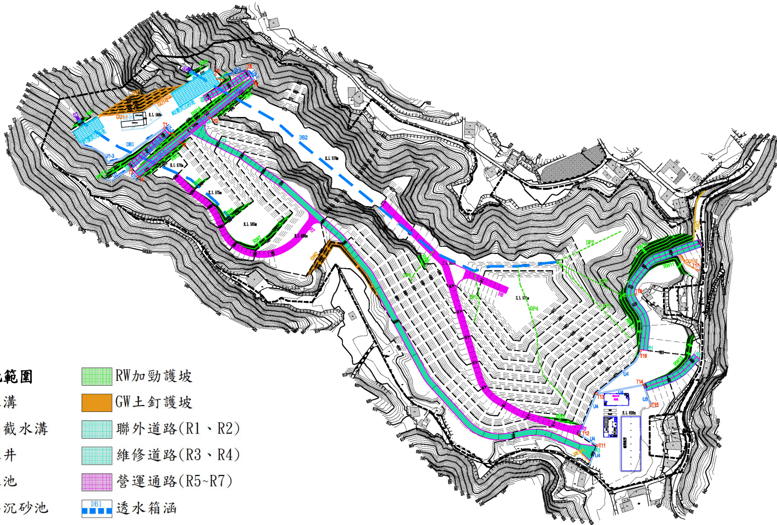
圖4-12 整地掩埋前地形配置圖
