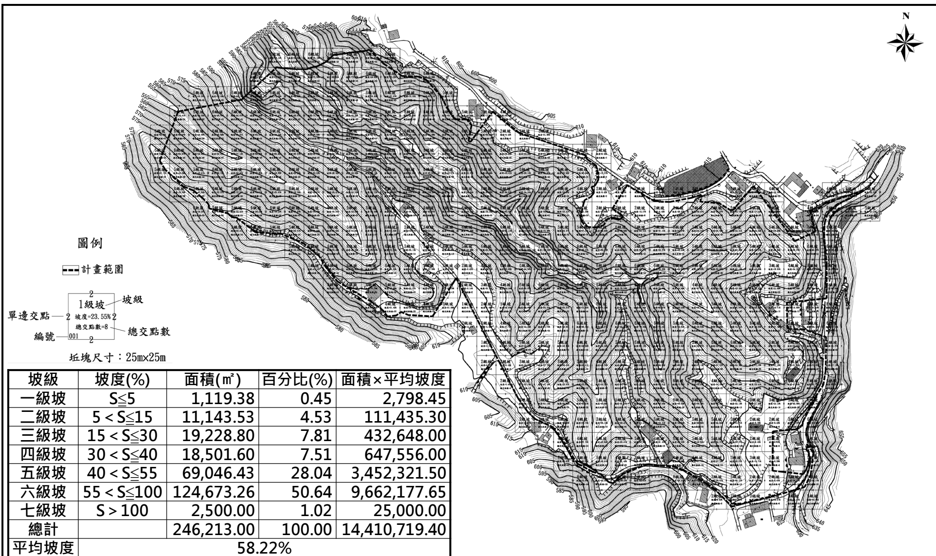
圖2-6 坡度分析圖
