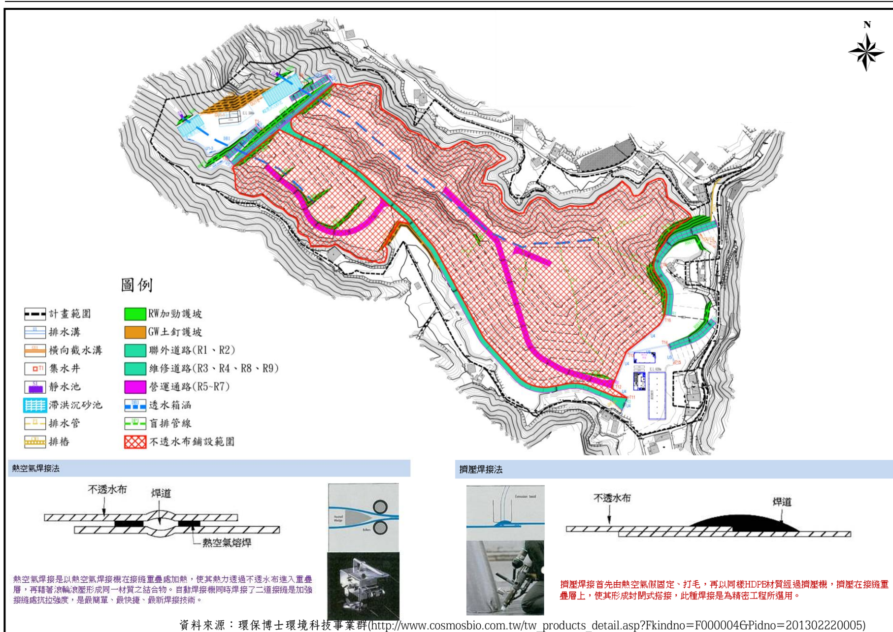
圖4-6 不透水及排水設施設計示意圖(一)
