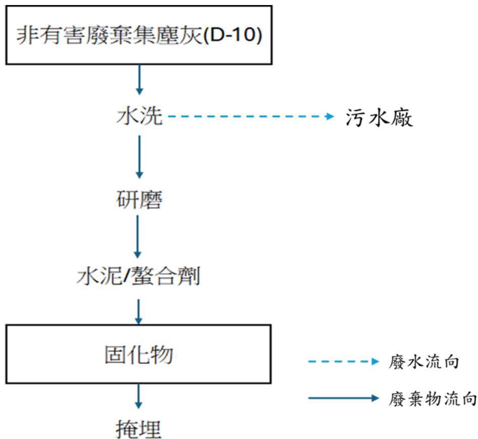
圖 4-9 固化流程示意圖
