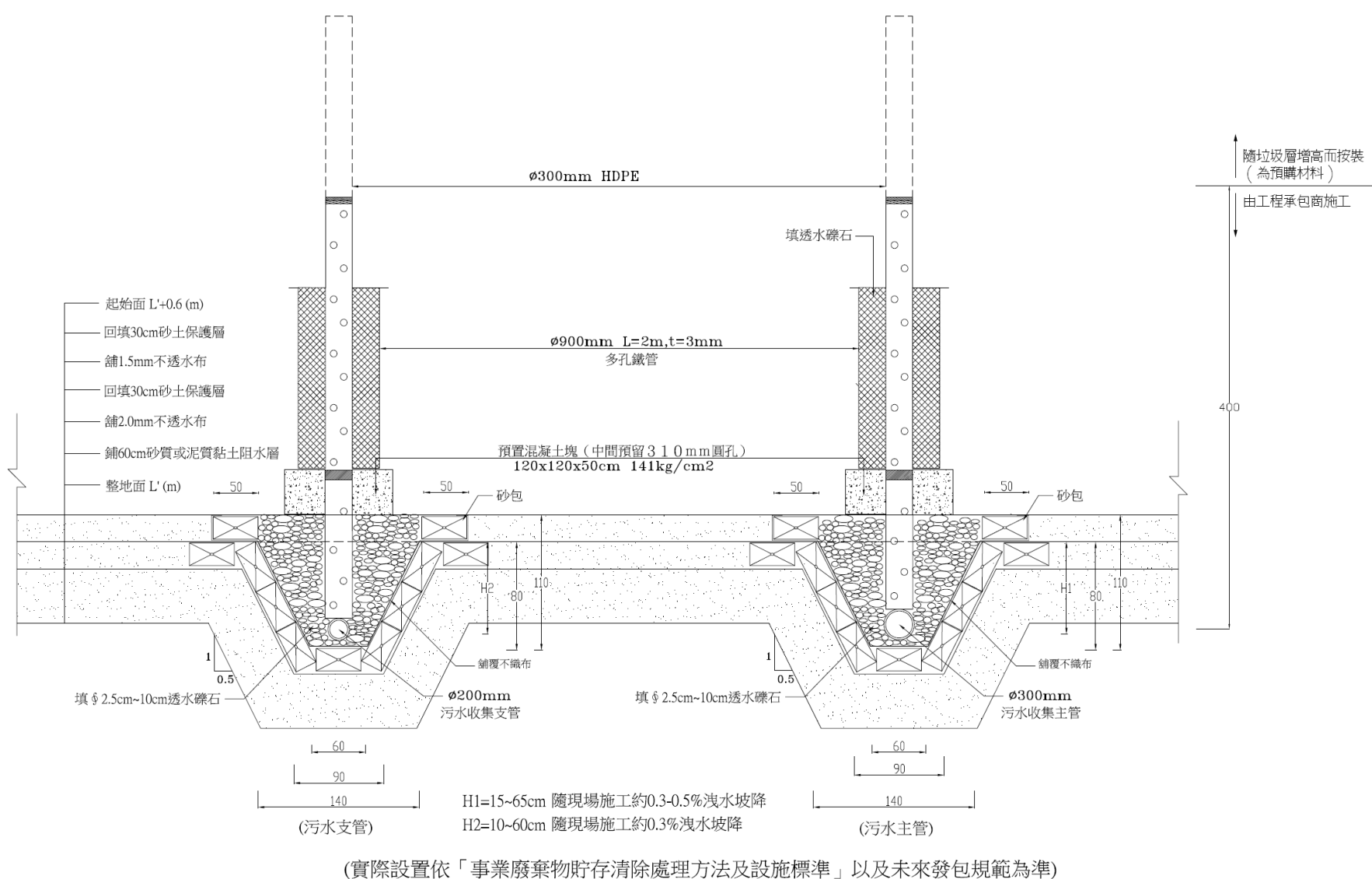
圖4-6 不透水及排水設施設計示意圖(二)
