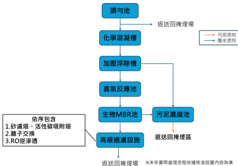
圖 5-1 廢污水處理流程圖
