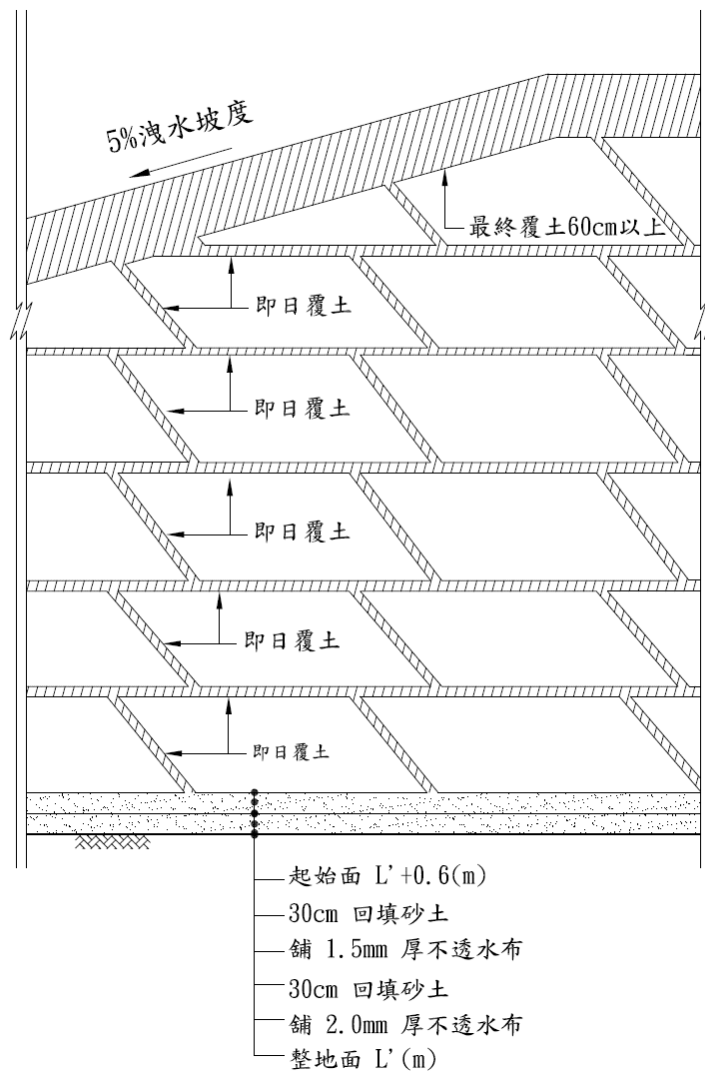
圖 5-9 最終覆土示意圖
