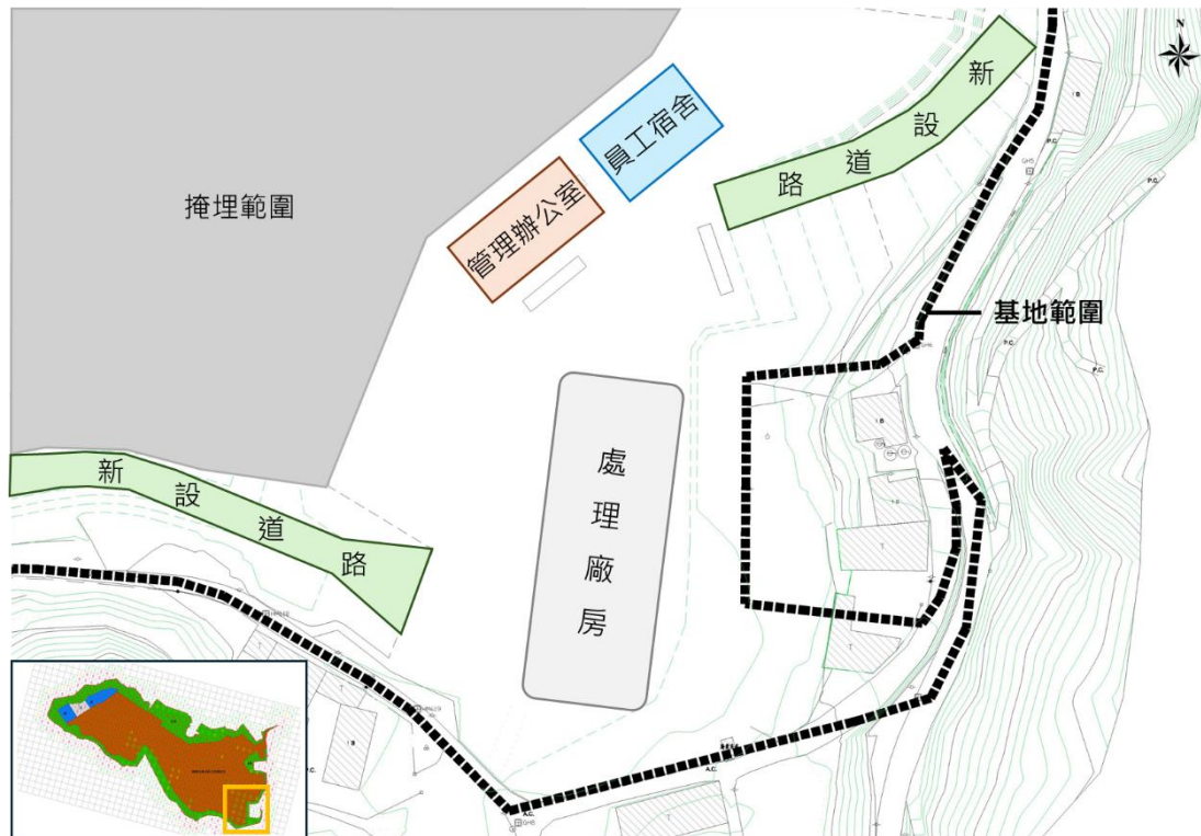
圖 4-10 建築位置示意圖
